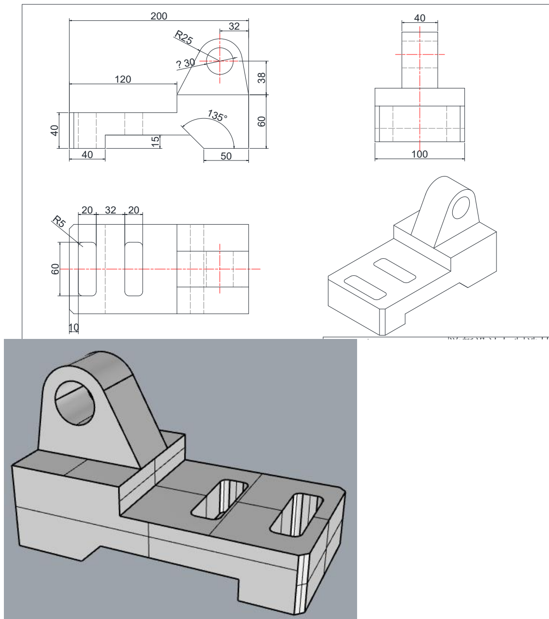
图 H2-13 底座创建
