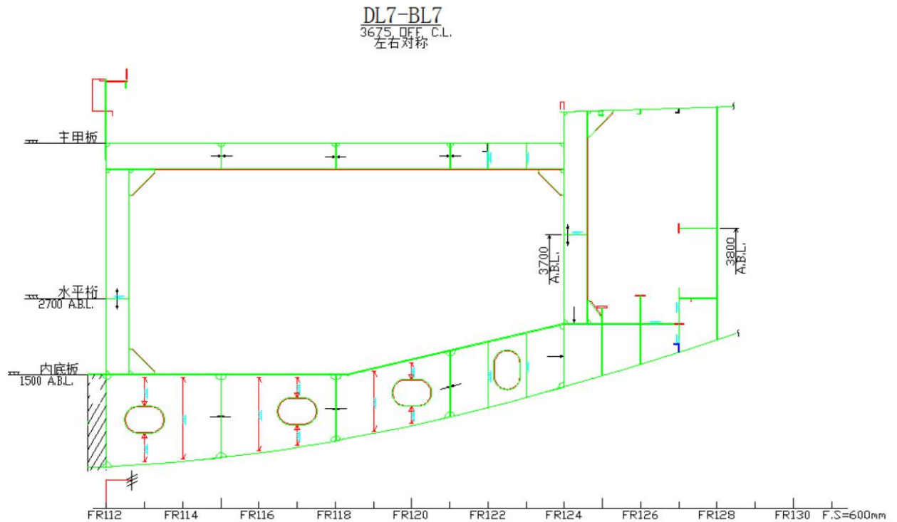
图 H2-12 某船体环段结构剖视图
