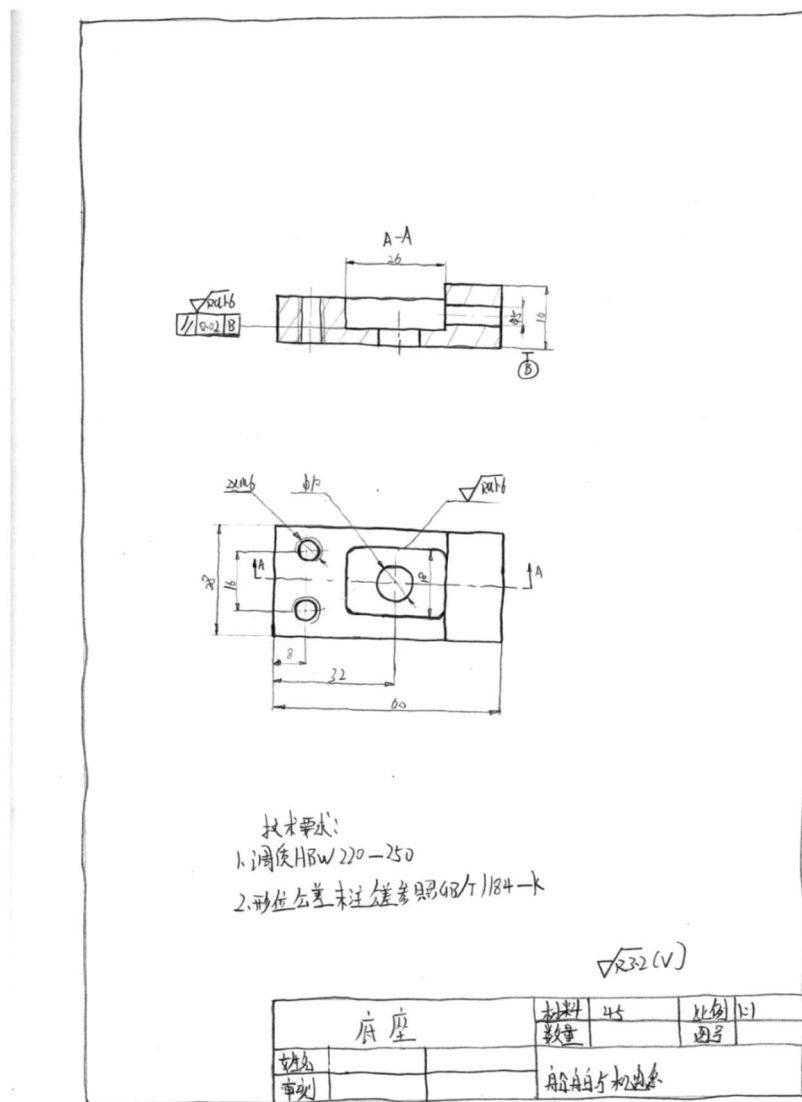
图 J1-3 底座
