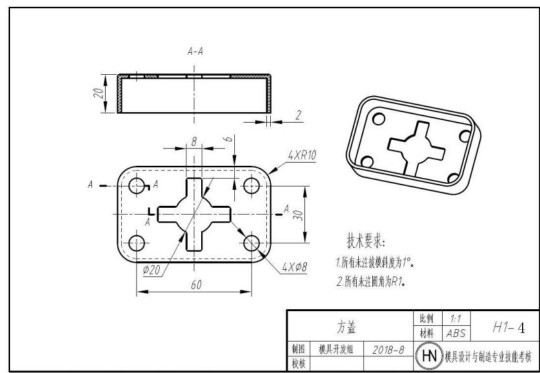
图 H1-4 方盖
