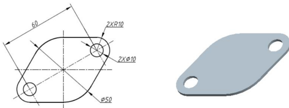
图 H2-8 斜形垫片
