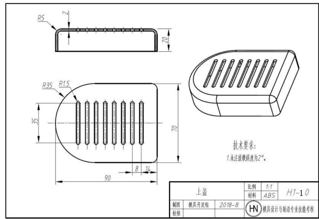
图 H1-10 上盖
