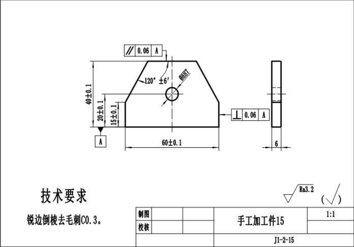
图T1-14 手工加工件 15
