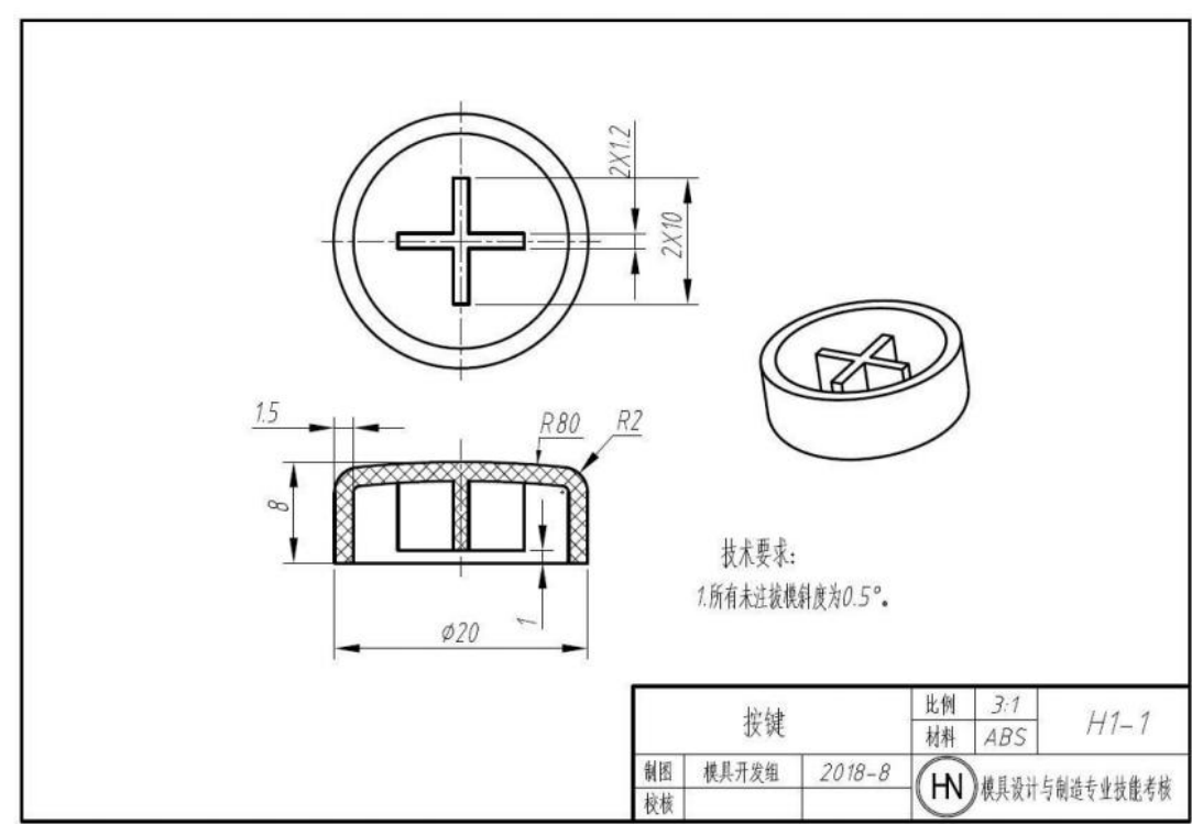
图 H1-1 按键
