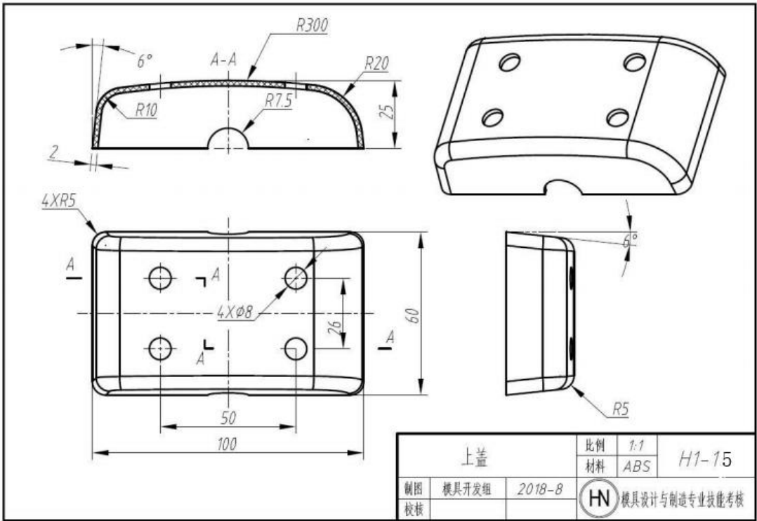
图 H1-15 上盖
