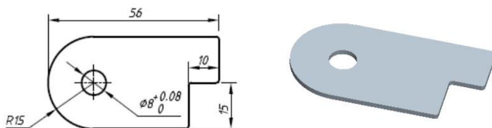
图 H2-5 电器零件
