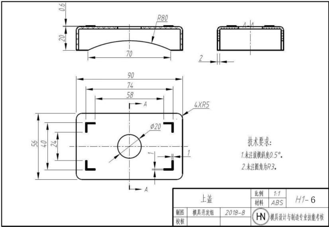
图 H1-6 上盖
