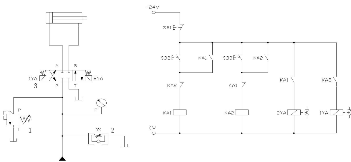
图 H1-2 回油路节流调速回路的液压回路和电气控制线路图
