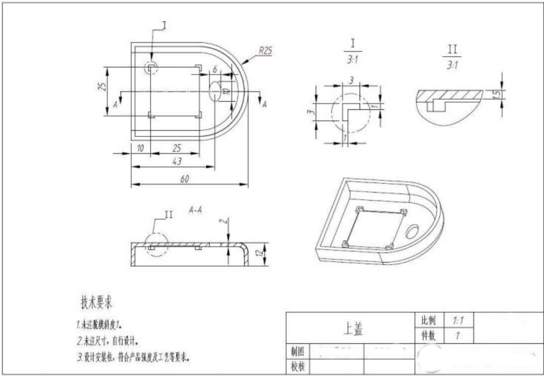
图 K1-1 上盖
