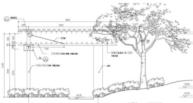
B 水树廊 (一) 侧立面图 1:30
