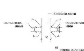
C 钢结构接点详图 1:10
