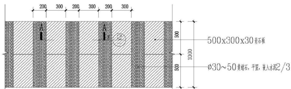
1 散步道铺装方式二 Scale 1:20
