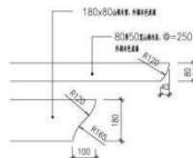
E 详图 1:10
