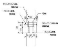
D 剖面图 1:10
