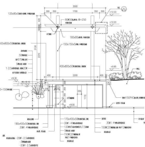
A 水树廊 (一) 剖面图 1:30
