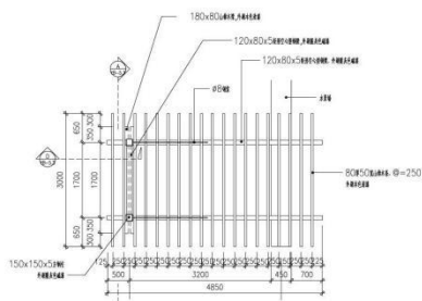
A 水树廊 (一) 顶平面图 1:50
