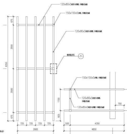
B 水树廊钢架平面图 1:50
