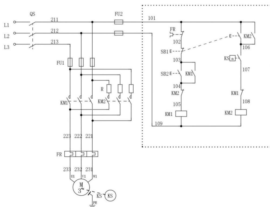
图 1-1-9 三相异步电动机单向启动及反接制动控制线路
