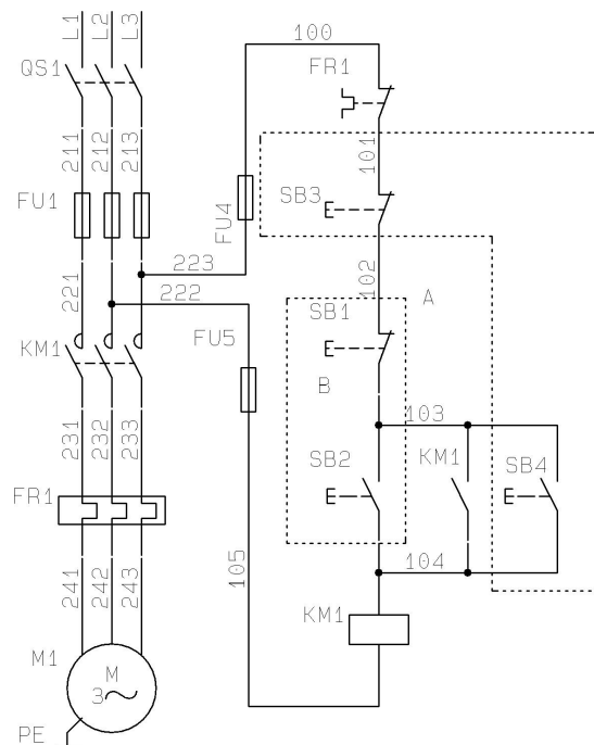
图 1-1-7 三相异步电动机两地控制线路
