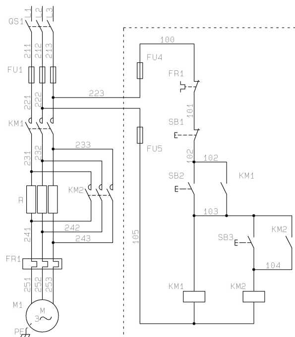
图 1-1-8 三相异步电动机串联电阻降压启动控制线路
