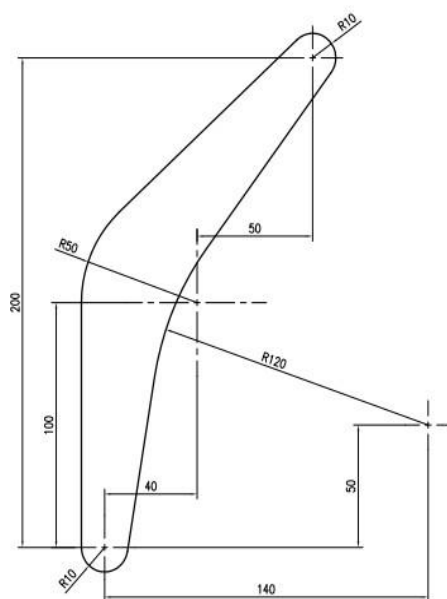
图 2-2-11 机器人运行轨迹平面尺寸图
