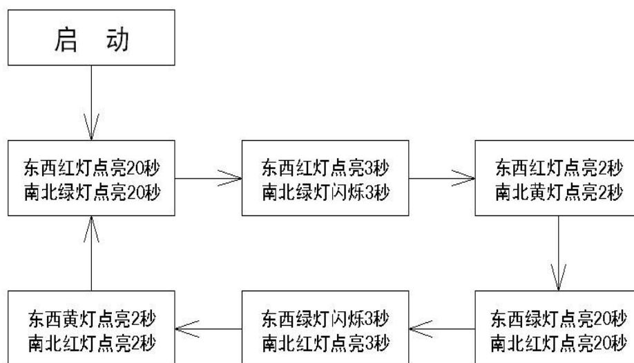
图2-1-12 十字路口交通灯控制要求
