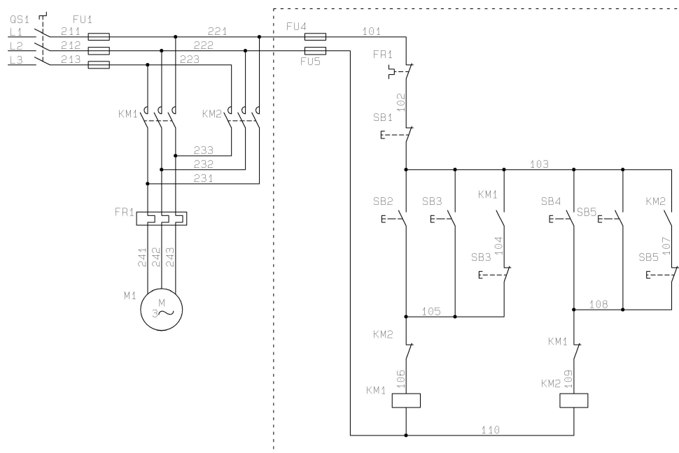
图 1-1-14 三相异步电动机的正反转带点动控制线路
