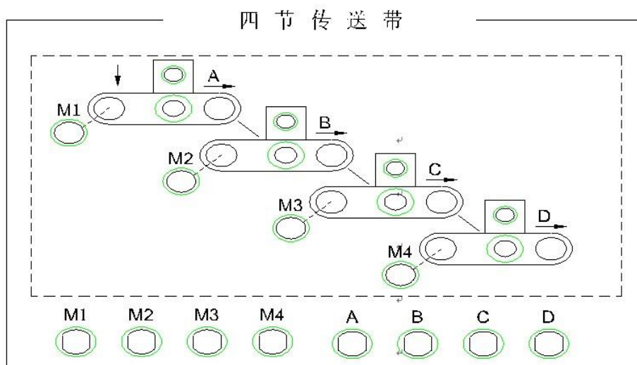
图2-1-11 四节传送带装置模拟示意图
