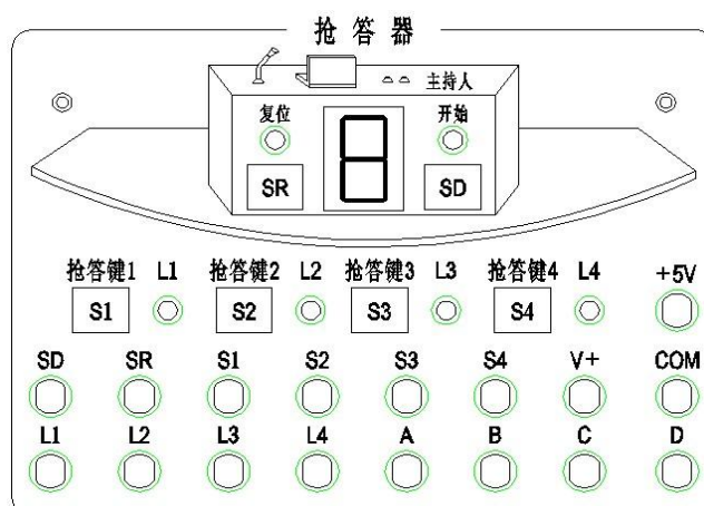
图2-1-13 抢答器示意图
