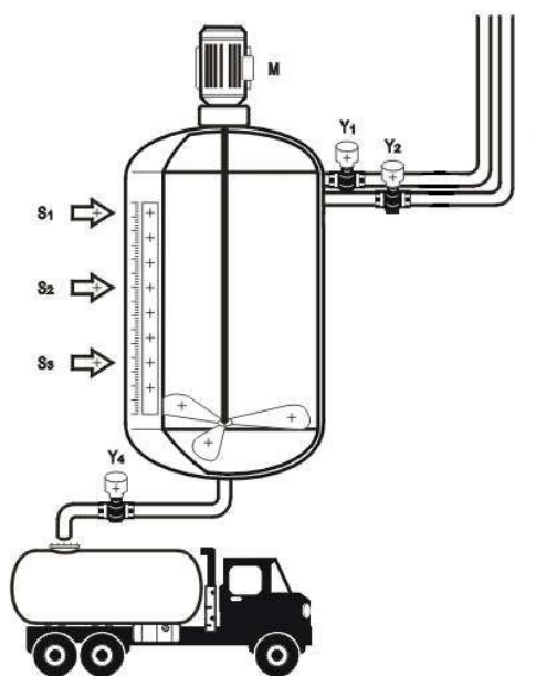
图2-1-10 多种液体自动混合示意模拟图
