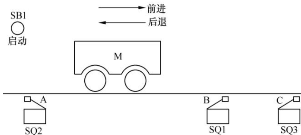
图2-1-15三点自动往返示意图
