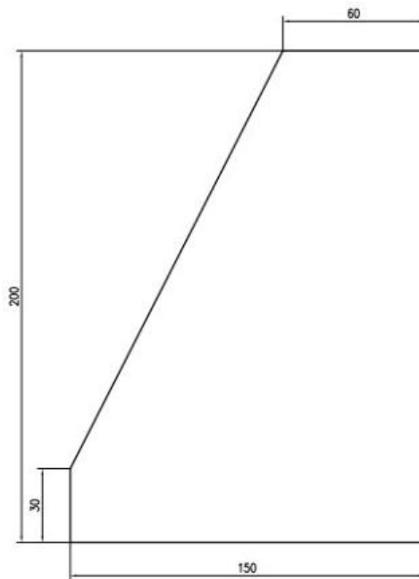
图 2-2-10 机器人运行轨迹平面尺寸图
