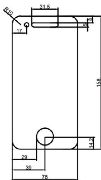
图 2-2-4 手机钢化玻璃膜平面尺寸图
