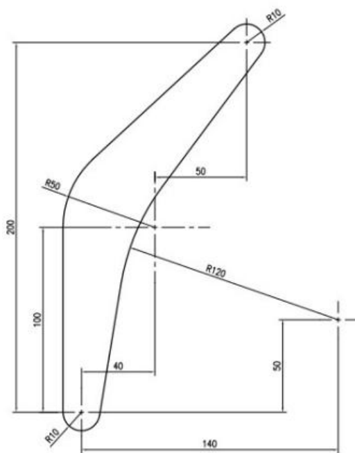
图 2-2-3机器人运行轨迹平面尺寸图
