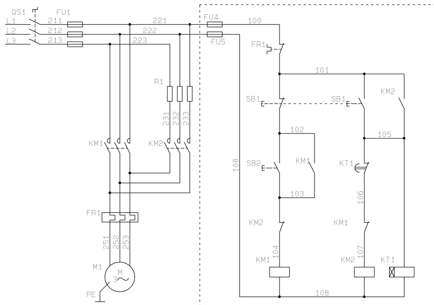
图 1-1-10 三相异步电动机单向启动及反接制动控制线路
