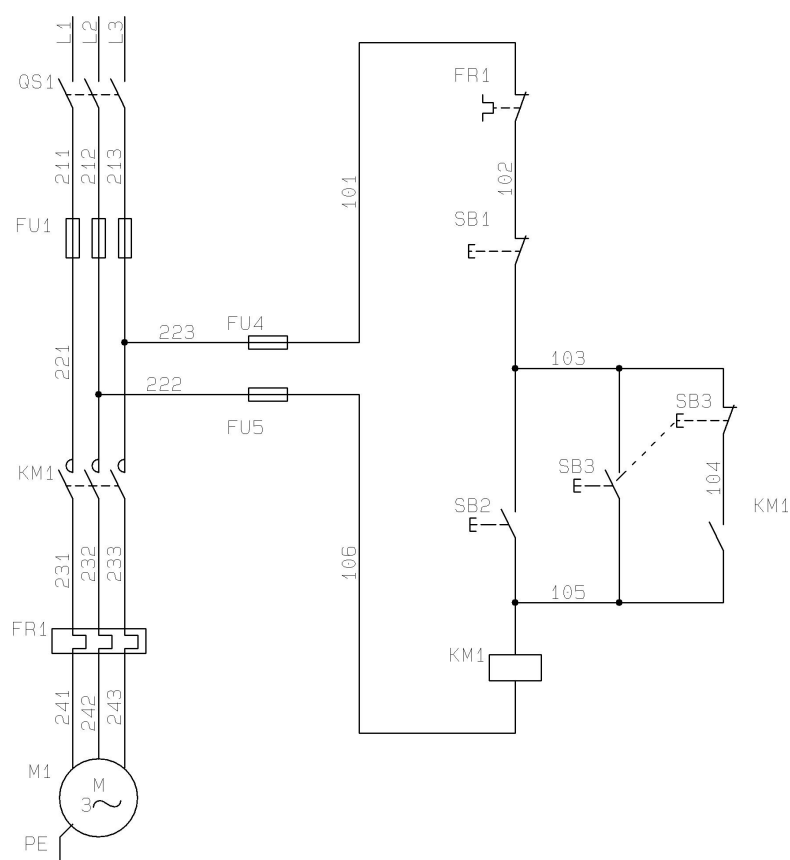
图 1-1-2 三相异步电动机点动和自锁控制线路
