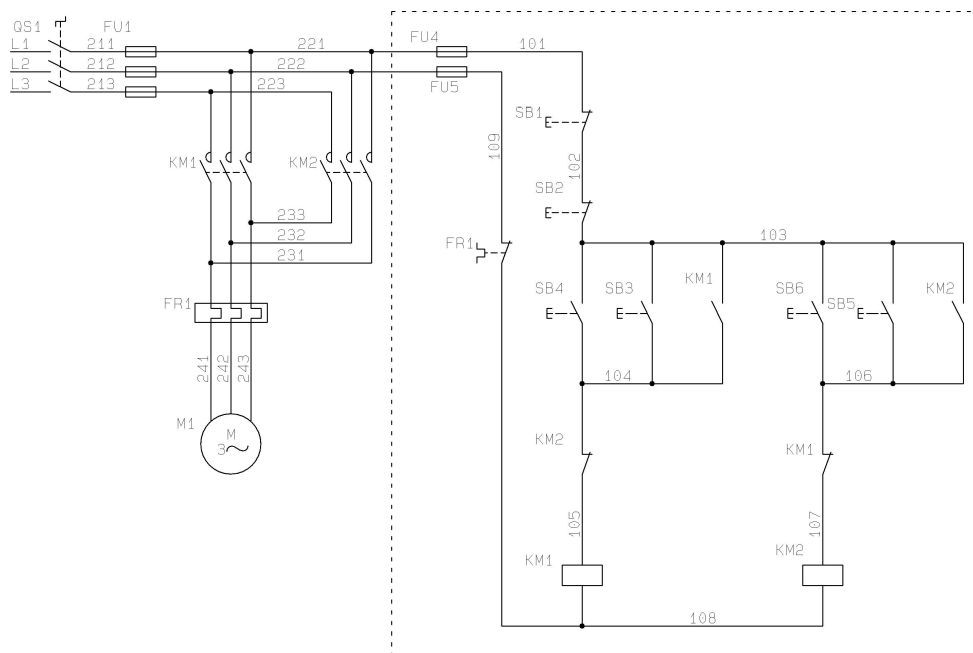
图 1-1-13 两地控制三相异步电动机的正反转控制线路
