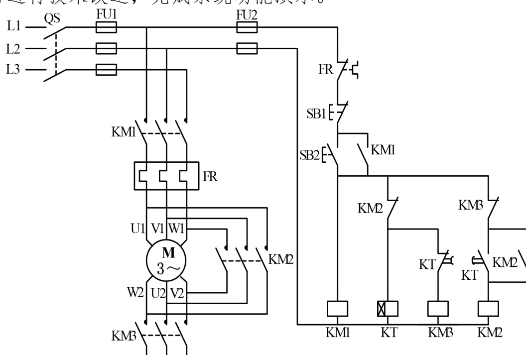
图2-1-1 时间继电器控制 Y— \Delta 降压启动控制线路图
