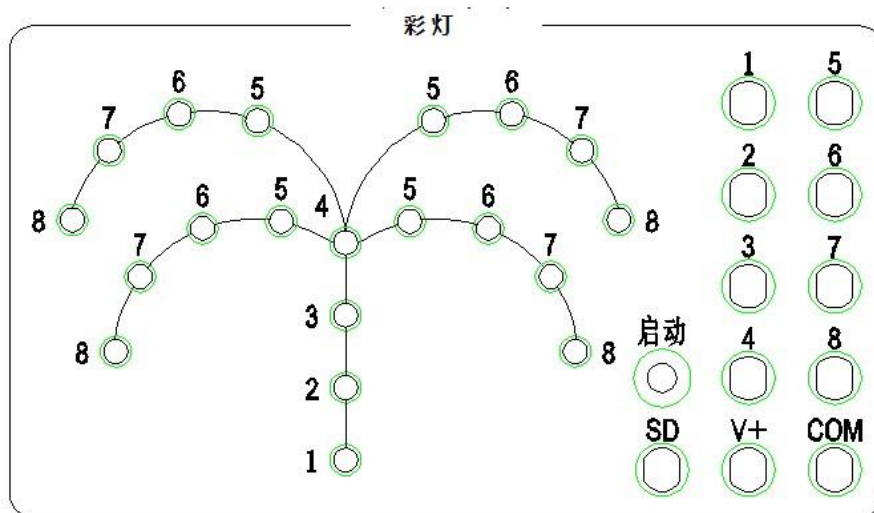
图2-1-9 彩灯控制面板示意图
