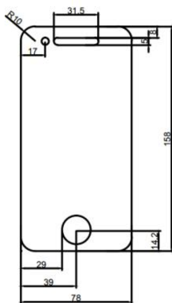
图 2-2-12 手机钢化玻璃膜平面尺寸图
