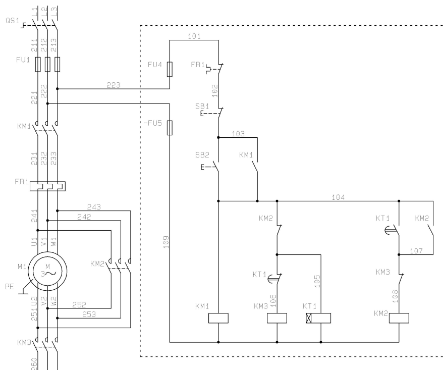
图 1-1-15 三相异步电动机的星三角降压启动控制线路
