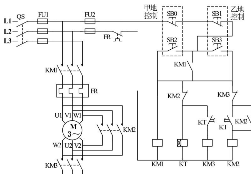
图2-1-4 两地控制的电动机Y—△降压启动控制线路
