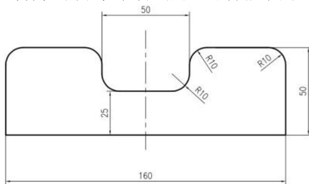
图 2-2-2 机器人运行轨迹平面尺寸图
