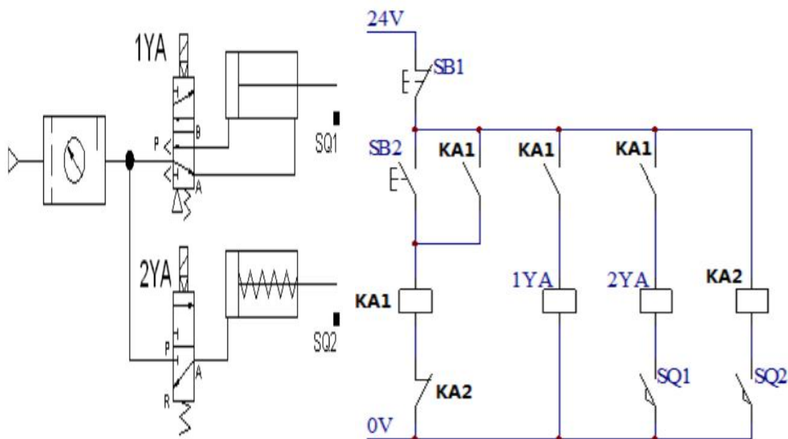
图2-1-8 双气缸顺序动作气动回路及电气控制线路图
