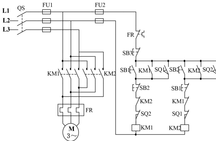
图2-1-2 电动机自动往返循环控制线路图
