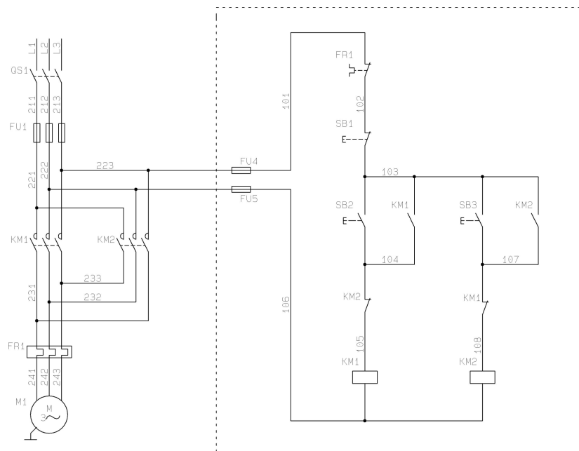
图 1-1-4 三相异步电动机的正反转控制线路
