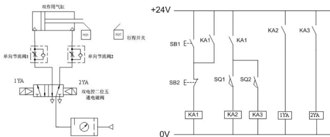
图2-1-6 单缸连续自动往返气动回路及电气控制原理图
