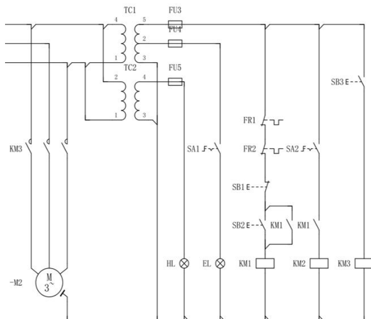
图2-1-5 C6140型车床电气控制线路
