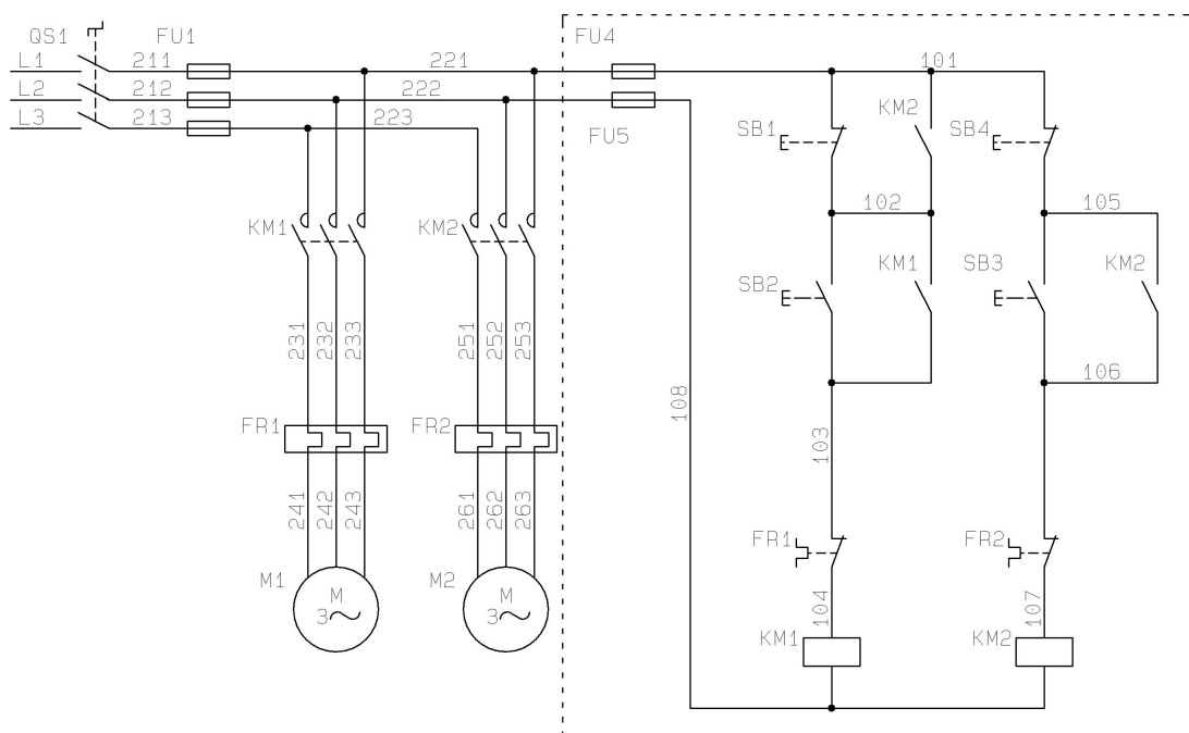
图 1-1-12 两台三相异步电动机顺序停止控制线路
