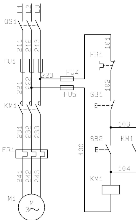
图 1-1-1 三相异步电动机启动停止线路
