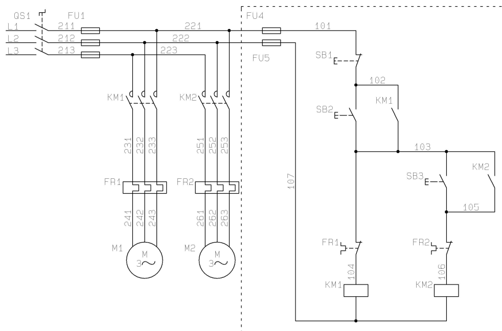
图 1-1-11 两台三相异步电动机顺序启动控制线路装调
